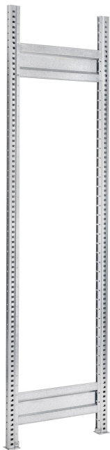
Skręcona rama regału
